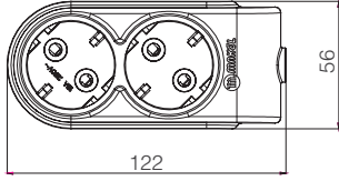
İkili Topraklı Grup Priz
