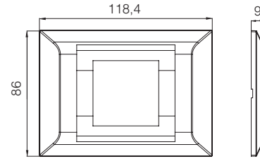
2M Çerçeve (3M Boyutunda)
