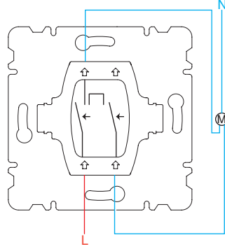
Jaluzi
