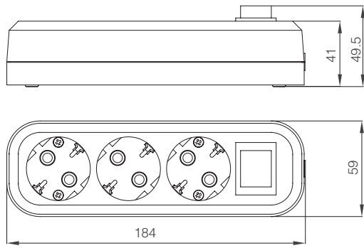
Üçlü Topraklı Grup Priz Anahtarı
