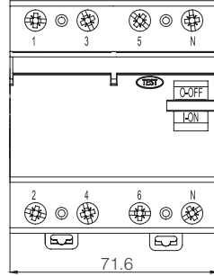
4 Kutuplu (RCCB) 6kA
