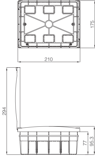
8'li Sıva Altı Klemensli Sigorta Kutusu
