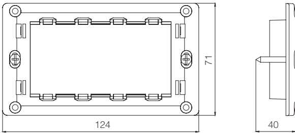
4M Karkas
