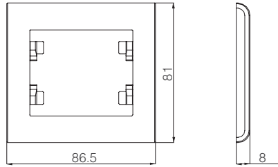
Tekli Çerçeve
