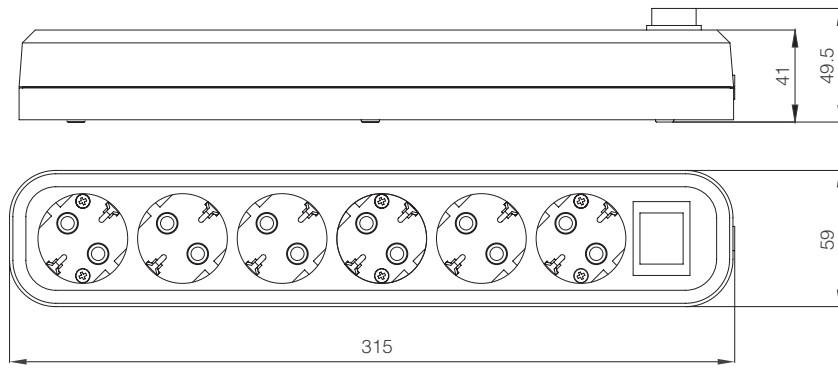
Altılı Topraklı Grup Priz Anahtarı
