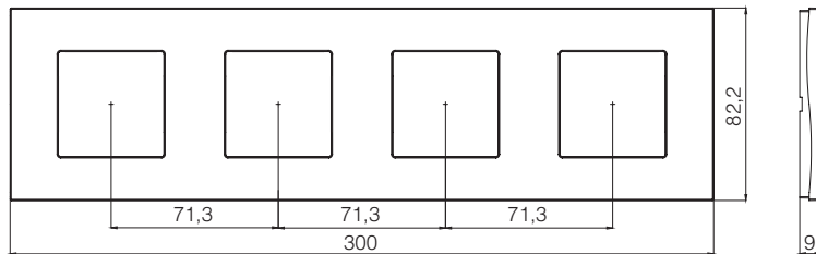
4X2M Çerçeve
