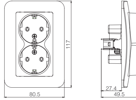
İkili Topraklı Priz
