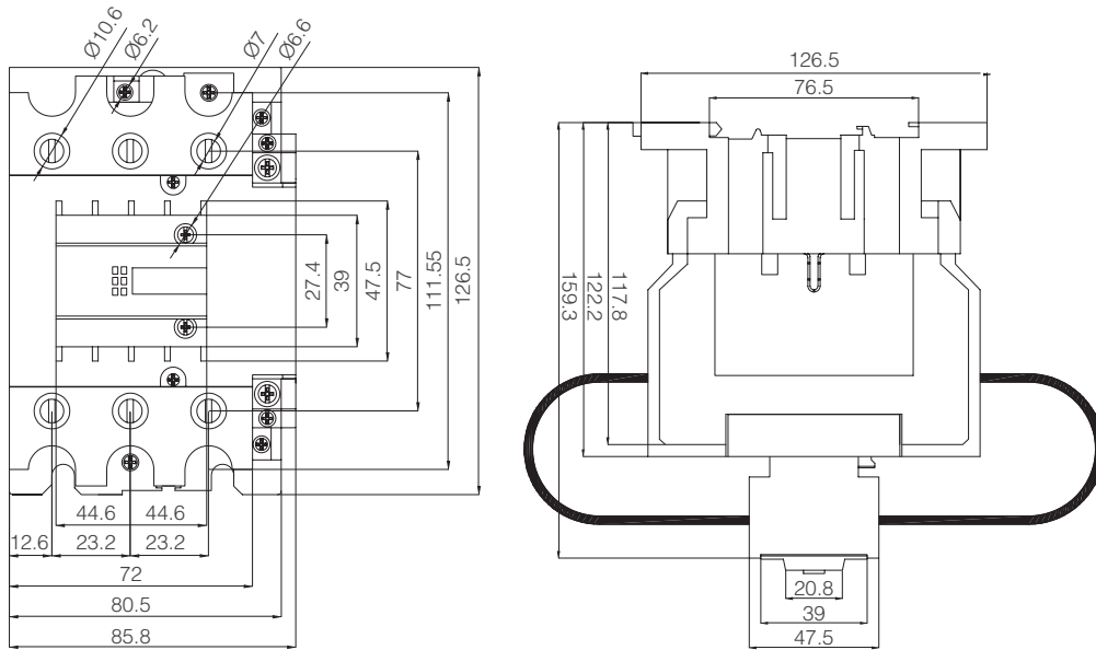
Kompanzasyon Kontaktörü 95A
