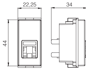
Numeris Priz (cat.3)
