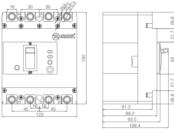
225 A Kaçak Akım Korumalı Kompakt Şalter
