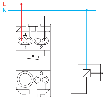
Kapı Otomatığı
