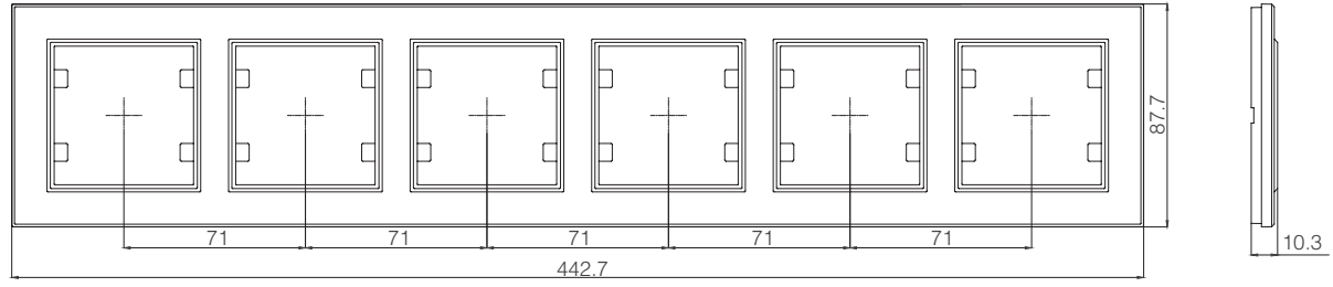
Altılı Yatay Çerçeve
