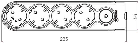
Dörtlü Topraklı Grup Priz Anahtarı
