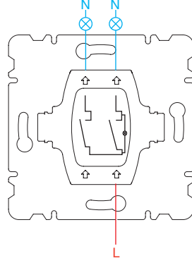
Işıklı Komütatör
