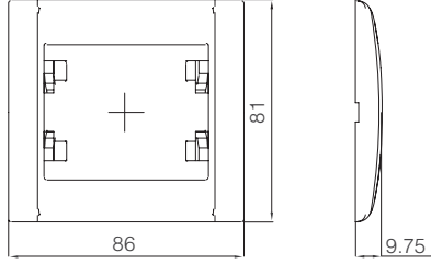
Tekli Çerçeve
