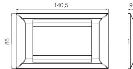
4M Çerçeve
