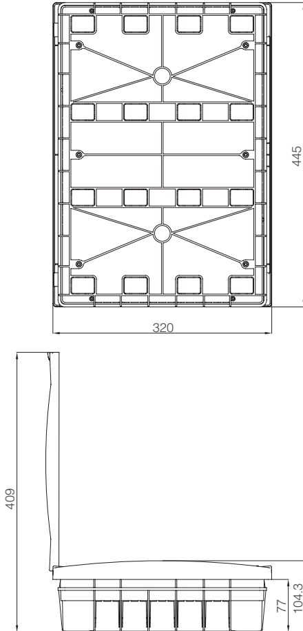
36'lü Siva Altı Klemensli Sigorta Kutusu Üç Katlı
