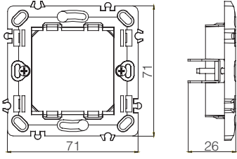
2M Karkas
