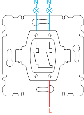
Komütatör
