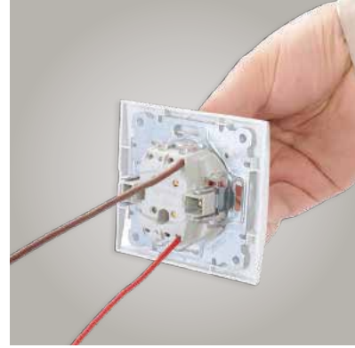
③ Soketli anahtarlarda kabloları iterek yuvalarına yerleştirin.
