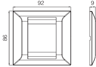
2M Çerçeve
