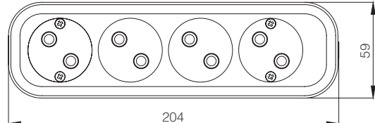
Dörtlü Grup Priz
