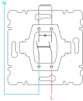
Uyarı Anahtarı
