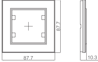
Tekli Çerçeve
