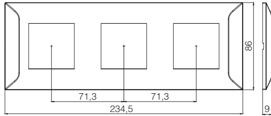
3X2M Çerçeve
