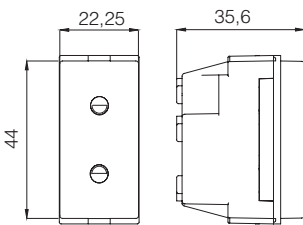
Cihaz Tipi Çocuk Korumalı Priz
