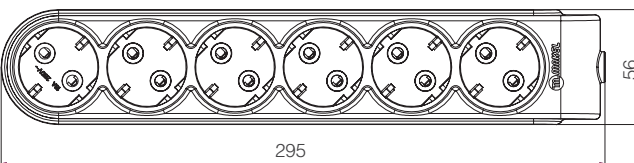
Altılı Topraklı Grup Priz
