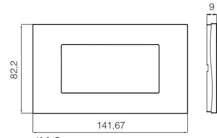
4M Çerçeve
