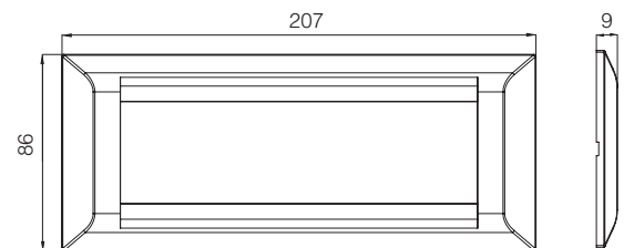
7M Çerçeve
