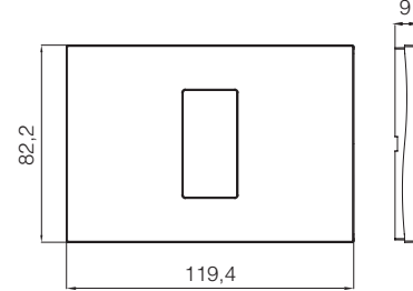
1M Çerçeve (3M Boyutunda)
