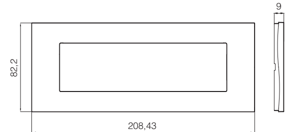
7M Çerçeve
