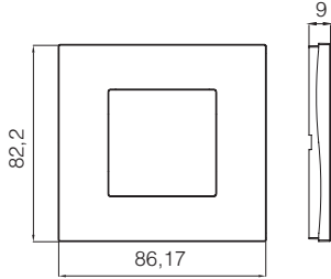
2M Çerçeve
