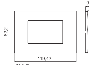
3M Çerçeve
