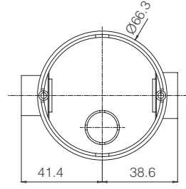
Sıva Altı Derin Kasa Geçmeli
