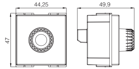
Bölgesel Ses Ayarı Paneli (BAP) 2M
