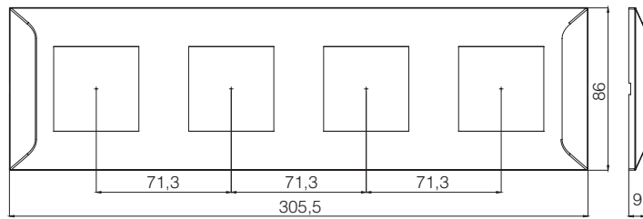
4X2M Çerçeve
