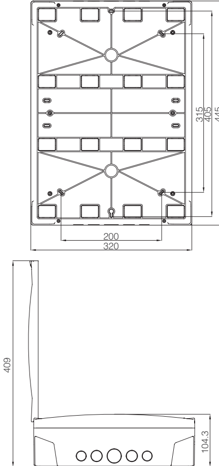
36'lü Siva Üstü Klemensli Sigorta Kutusu Üç Katlı
