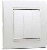
Üçlü Anahtar 3 Tuşlu (3+3) 3 Giriş, 3 Çıkış 31002092 10 AX, 250 V~ EN 60669-1 Kutu / Koli Adedi - 12 / 120
