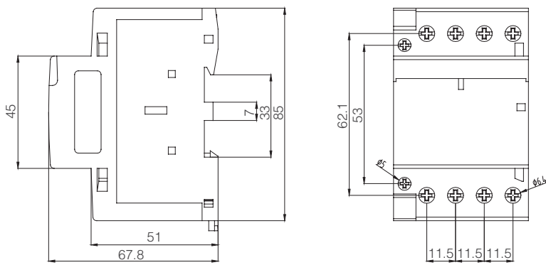
KNHC-40-63 Modüler Kontaktör 40-63A 230V AC 4Kutuplu 4NO-2NO+2NC-4NC-3NO+1NC-3NC+1NO
